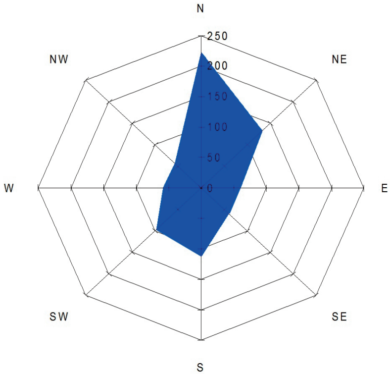
Figura 6: Frecuencia media anual de direcciones del viento entre serie 1941 y 2011
